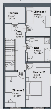
Grundriss - TYP A Obergeschoss - 69,77 m 2
