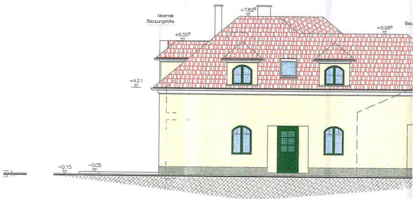
Westansicht 1:100
