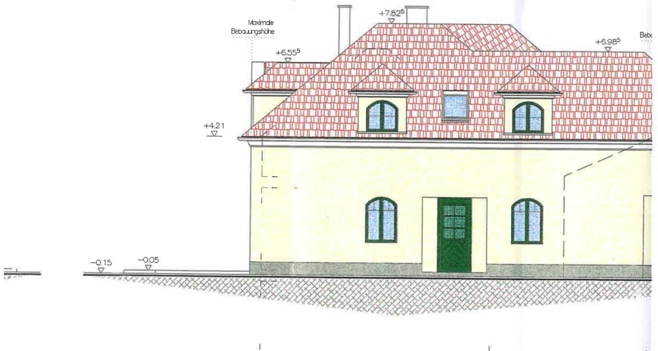
Westansicht 1:100
