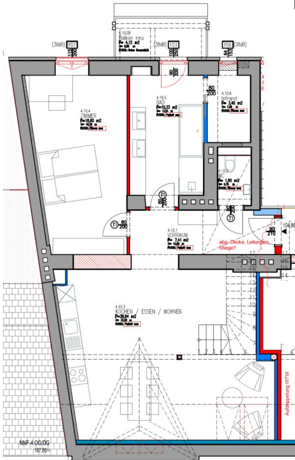
Planskizze 4. OG Variante 2
