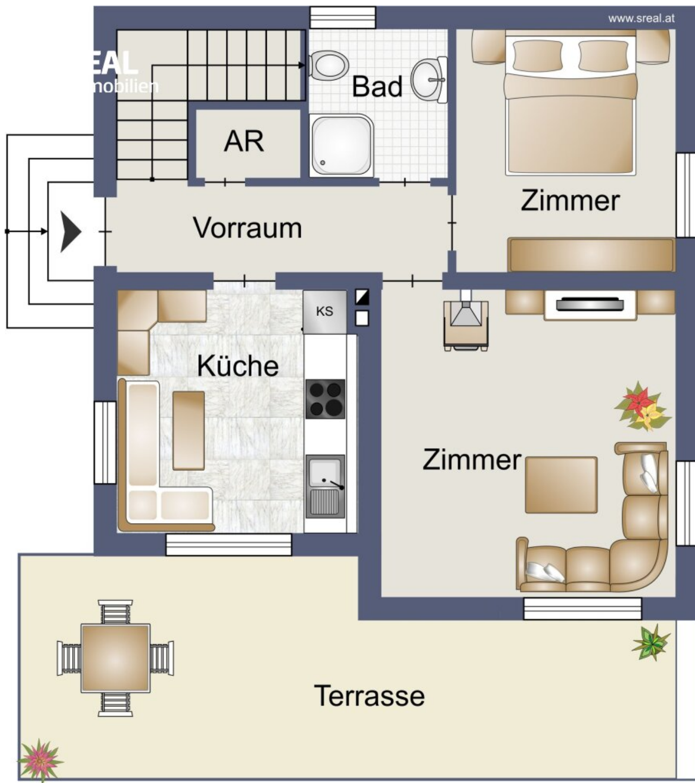
Skizze Erdgeschoss
