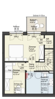
Obergeschoß
