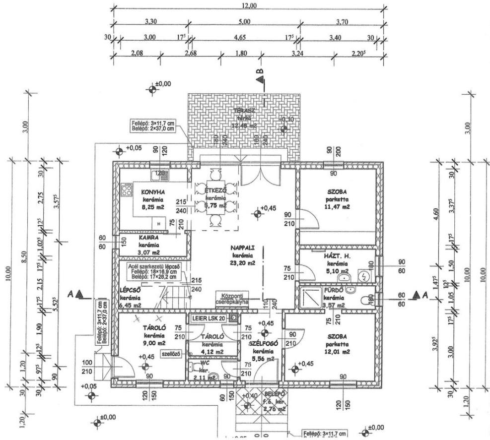
FÖLDSZINTI ALAPRAJZ M 1:100
