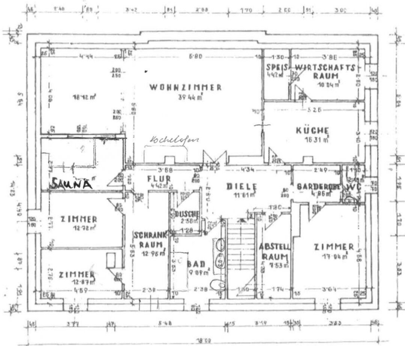
GRUNDRISS Dachgeschoß
