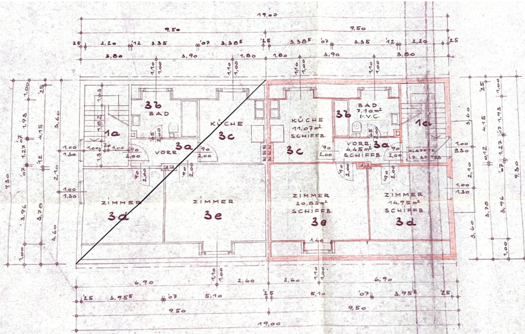
DACHGESCHOSS III
