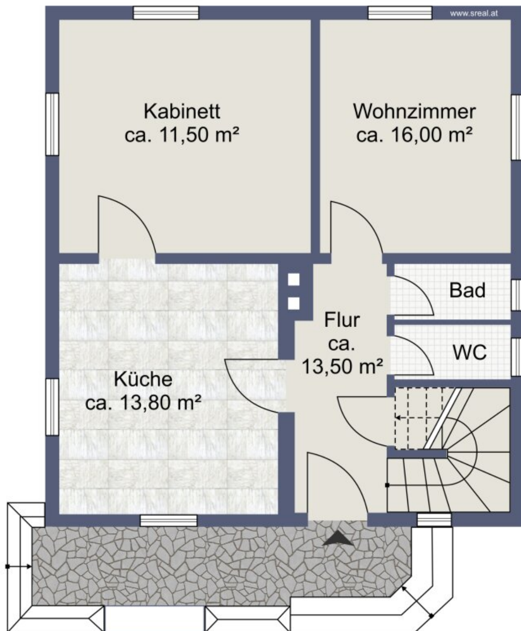
Skizze Erdgeschoss
