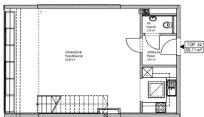
1. DACHGESCHOSS
