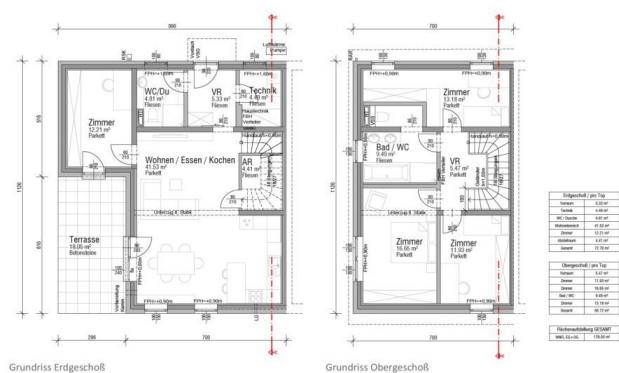
Grundrisse - Doppelhäuser Einöd
