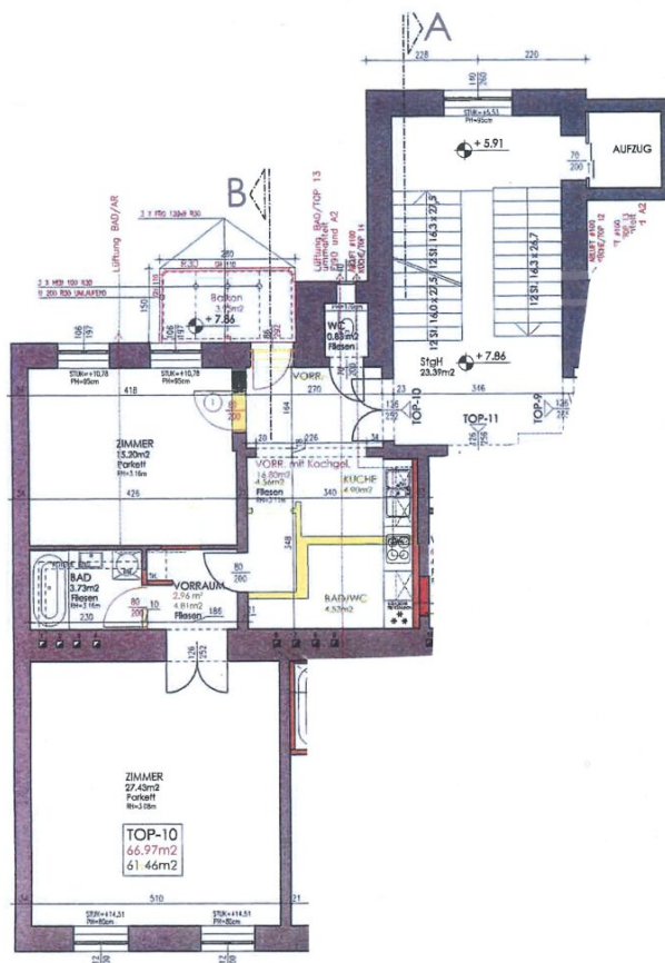
2. OBERGESCHOSS
