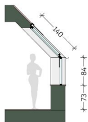
Schnitt 1:50 Dachschräge
