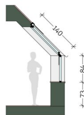
Schnitt 1:50 Dachschräge
