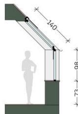
Schnitt 1:50 Dachschräge
