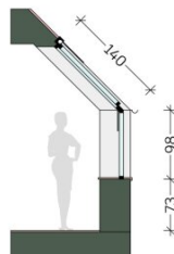
Schnitt 1:50 Dachschräge
