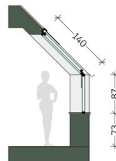
Schnitt 1:50 Dachschräge
