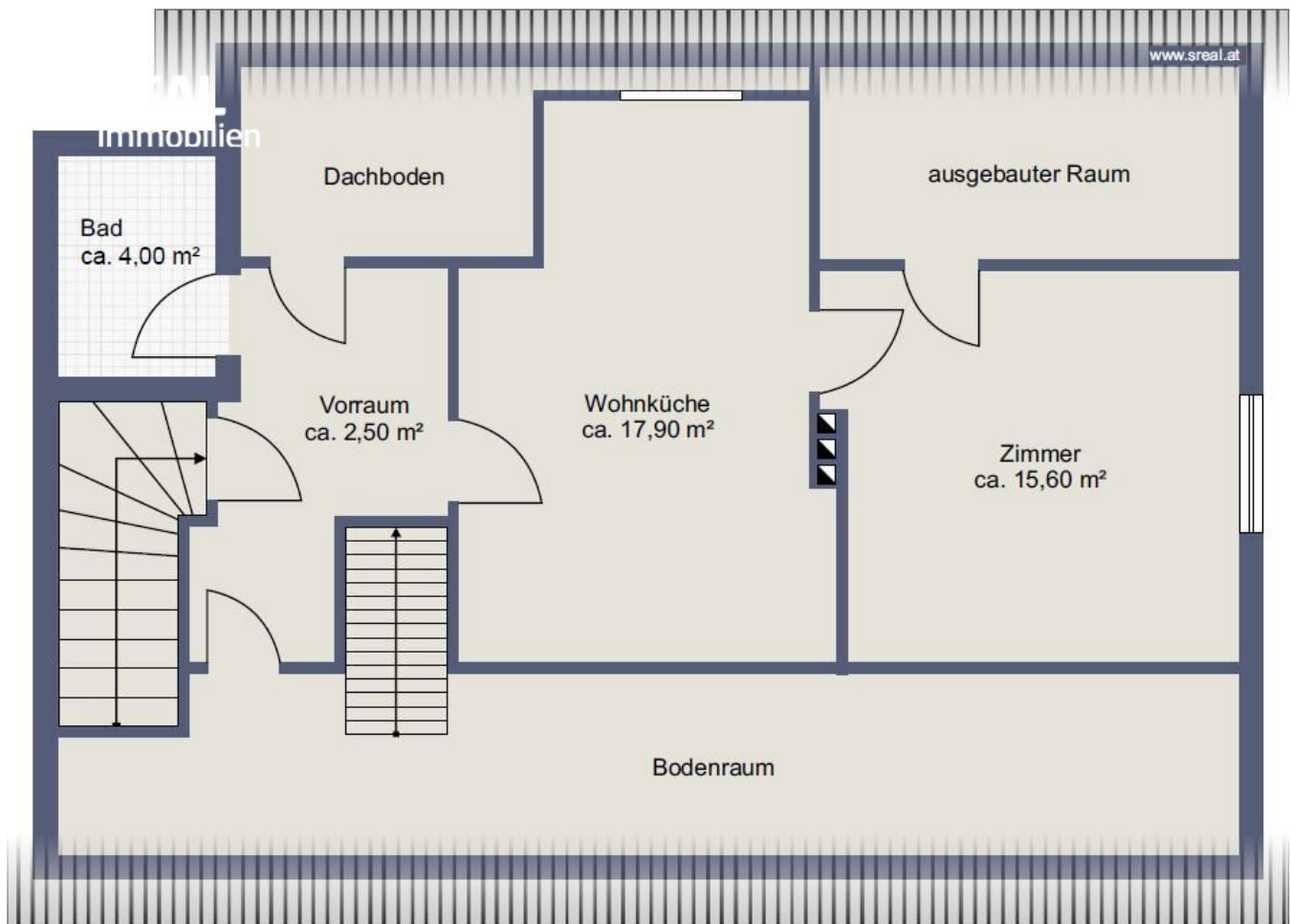
Planliche Darstellung Dachgeschoss
