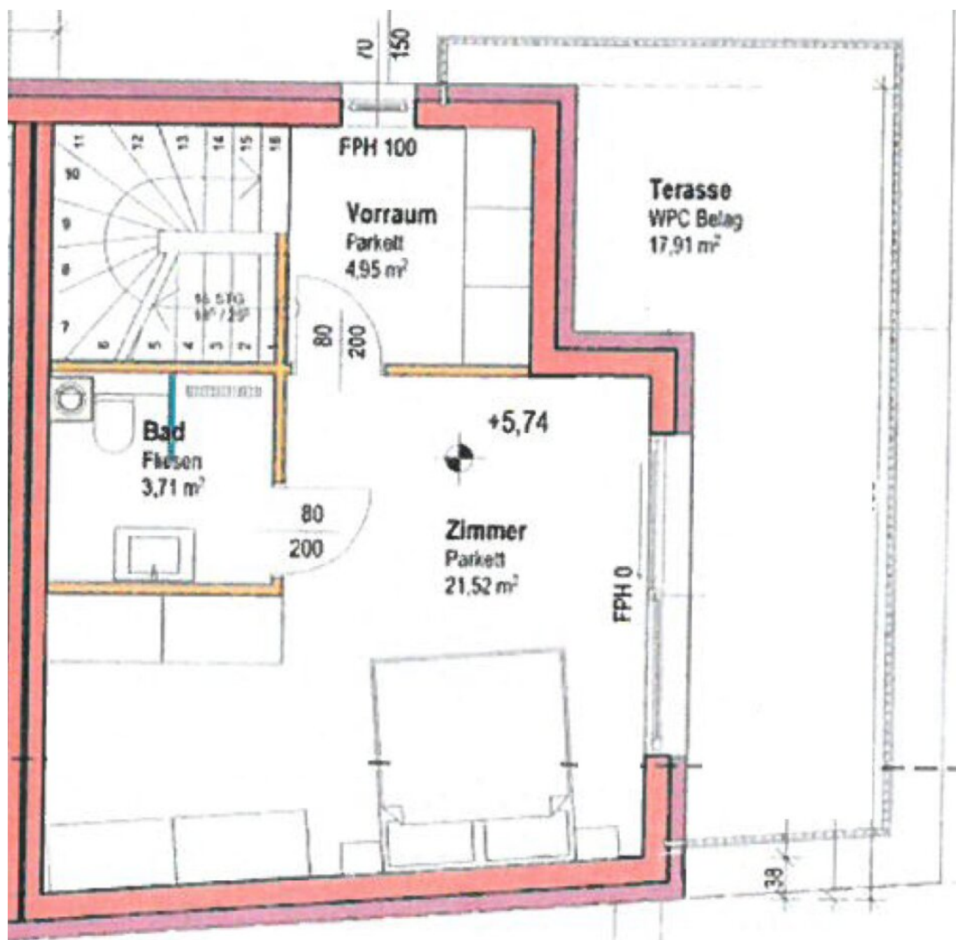
DACHGESCHOSS
