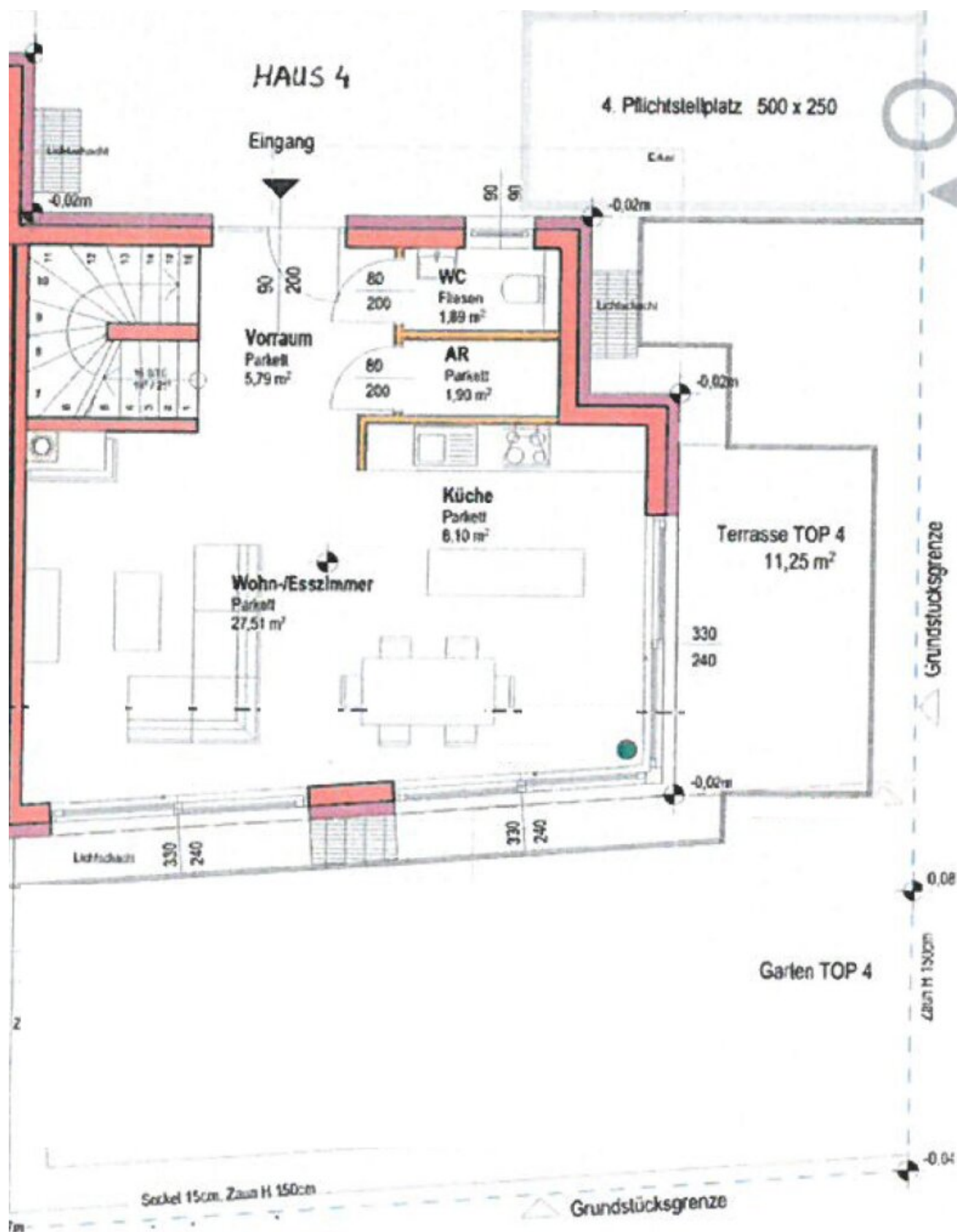
ERDGESCHOSS
