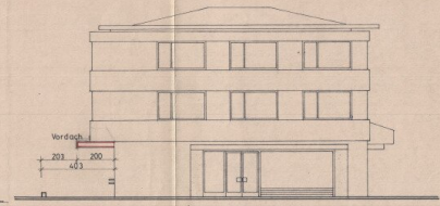
OSTANSICHT 1:100 (STRASSENANSICHT)
