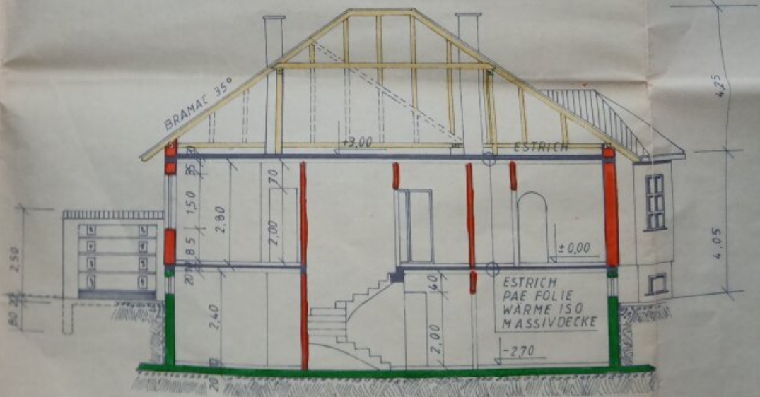
SCHNITT A-B
