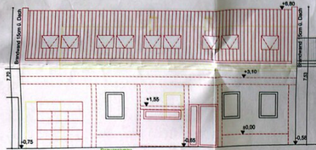
WESTANSICHT(STRASSE)
