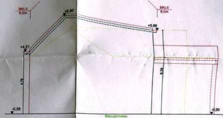
SÜDANSICHT
