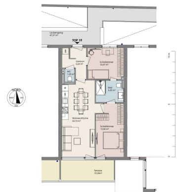
GRUNDRISS TOP 19
