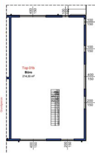
Grundrissausschnitt Zwischenebene Top 1b M 1:200
