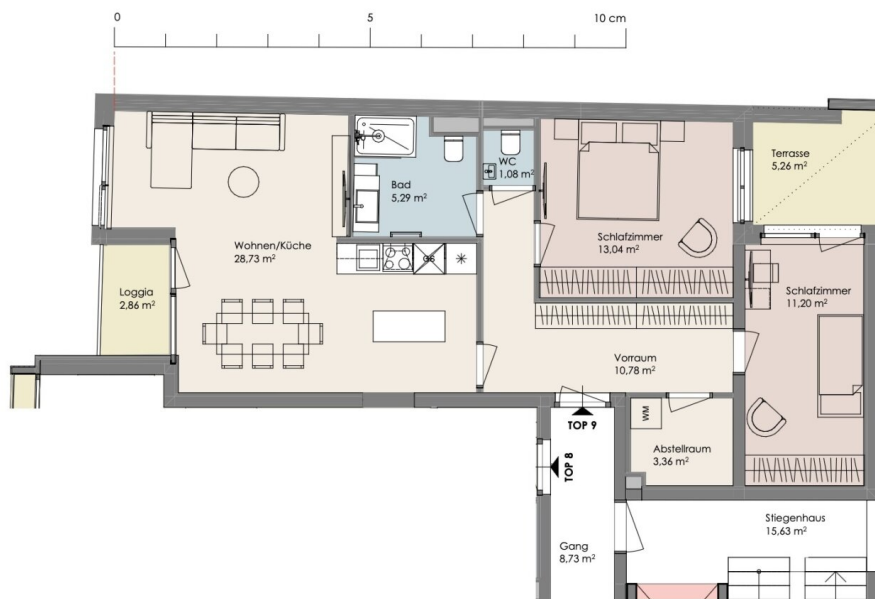
GRUNDRISS TOP 9
