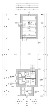
Kellergeschoss
