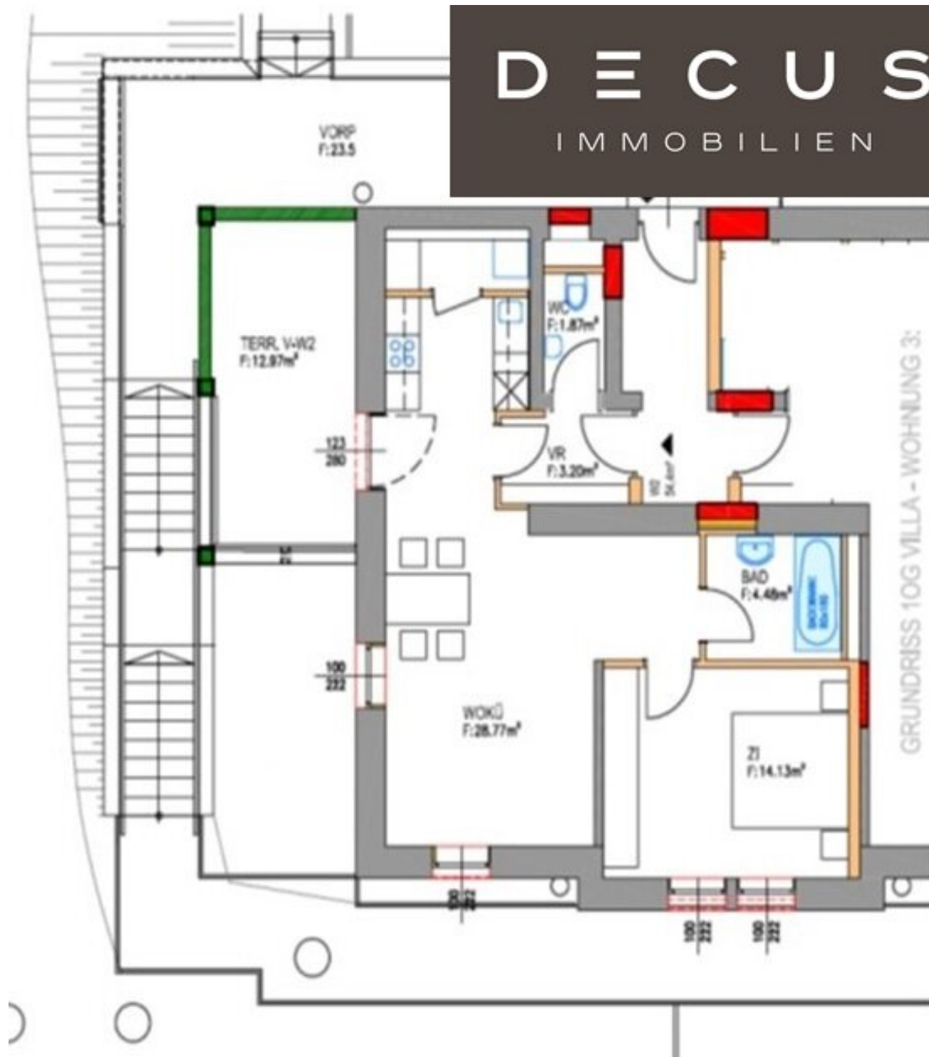
GRUNDRISS 1.OBERGESCHOSS :
