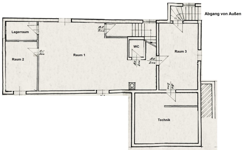
Grundriss-Skizze Untergeschoss
