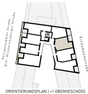
ORIENTIERUNGSPLAN | +1 OBERGESCHOSS
