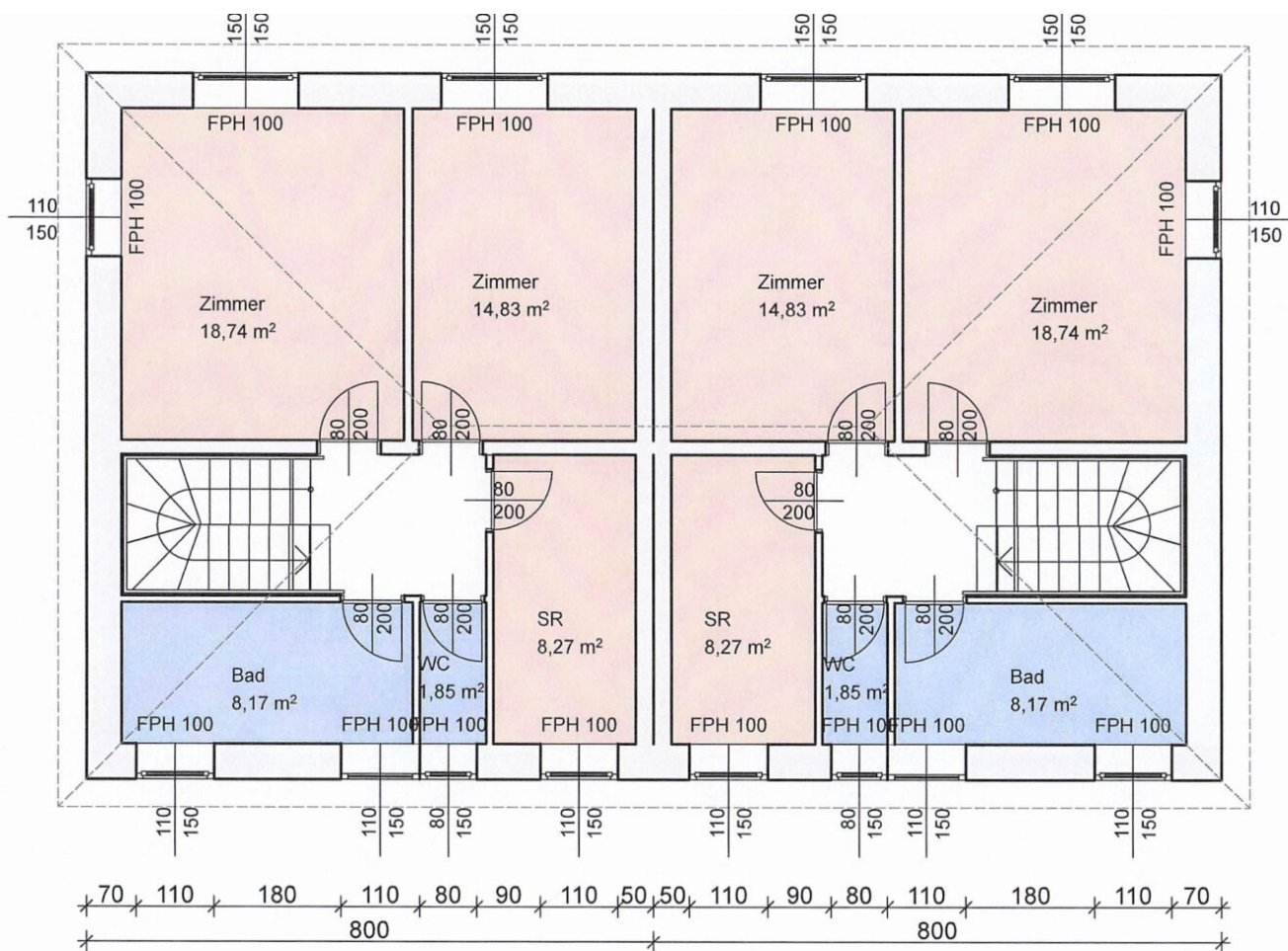
Obergeschoß Maßstab 1:100
