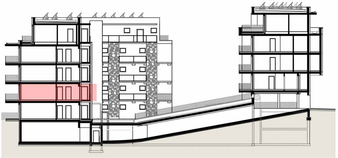
SYSTEMSCHNITT M 1:500
