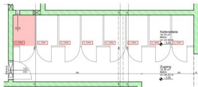
Planausschnitt KELLERGESCHOSS - Abteil TOP 08 - WEST Planstand = Ausführungsplan M: 1:100
