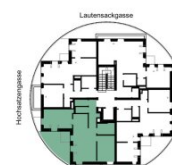
GESCHOSSPLAN
