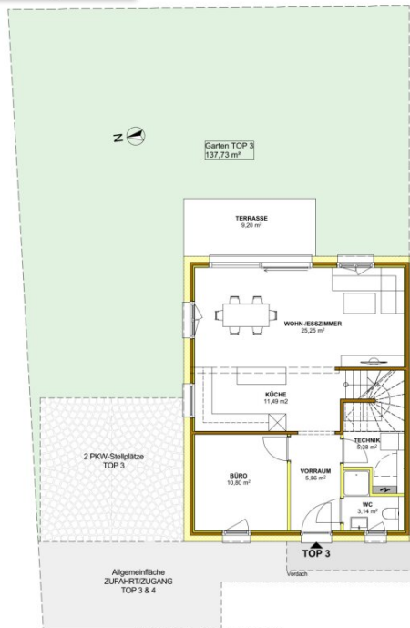
ERDGESCHOSS
