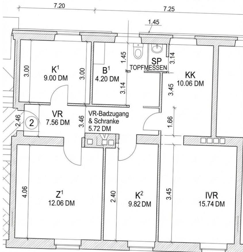
Umbauprojekt - Grundriss OG - Maßstab 1:50
