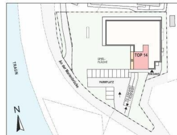
LAGEPLAN M1:1000
