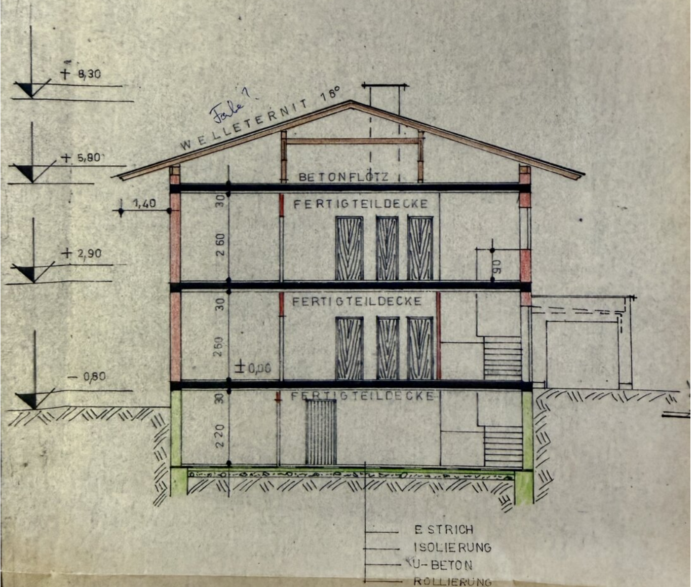
SCHNITT A-B
