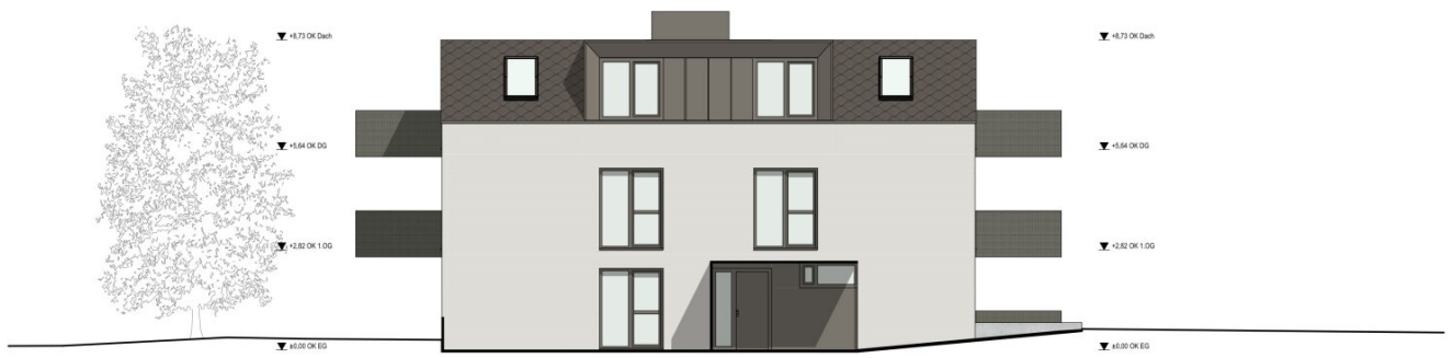
ANSICHT NORD
