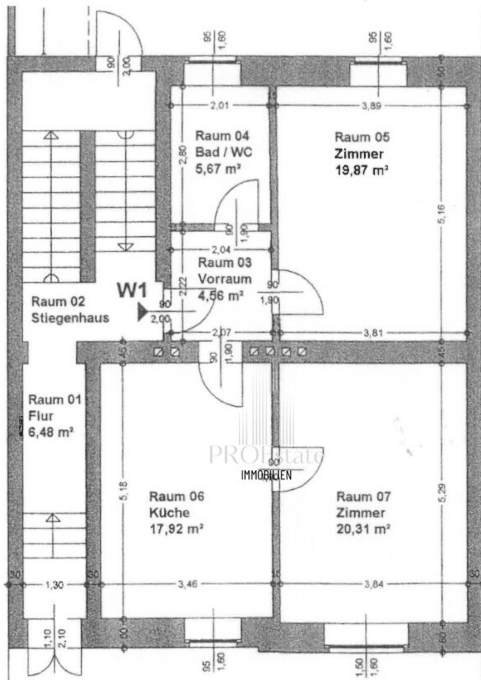
Grundriss - EG
