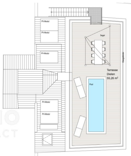
DACHDRAUFSICHT
