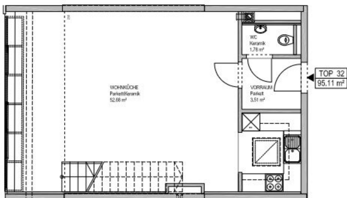
1. DACHGESCHOSS
