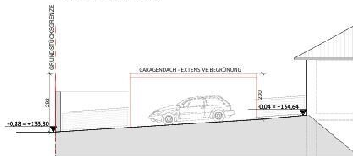
SÜD-WEST ANSICHT
