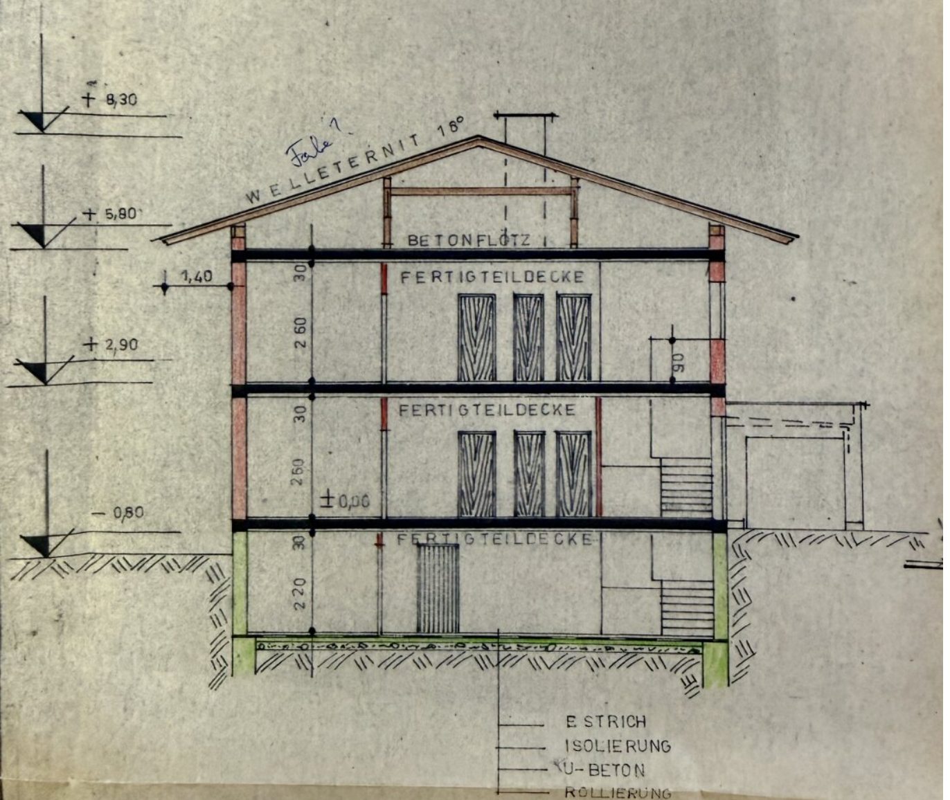
SCHNITT A-B
