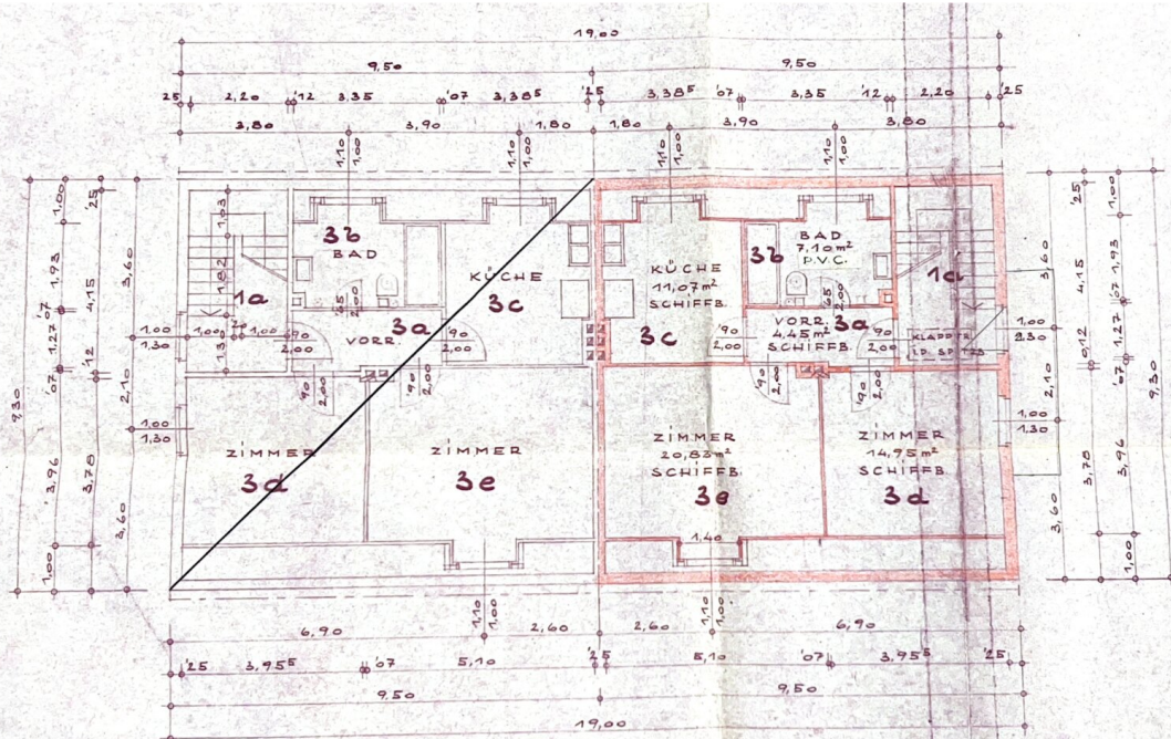
DACHGESCHOSS III
