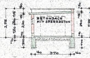
QUERSCHNITT
