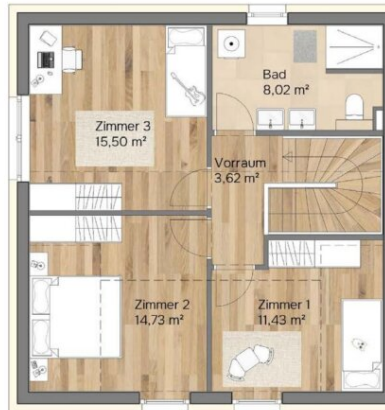
Obergeschoss Raumhöhe 1,75-3,50 m
