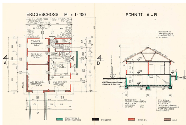
Einreichplan April 1971
