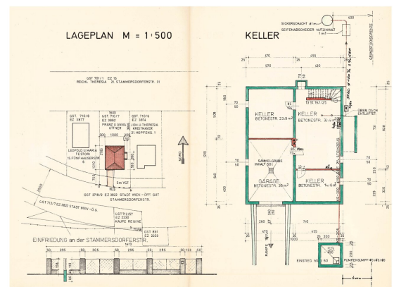
Einreichplan April 1971
