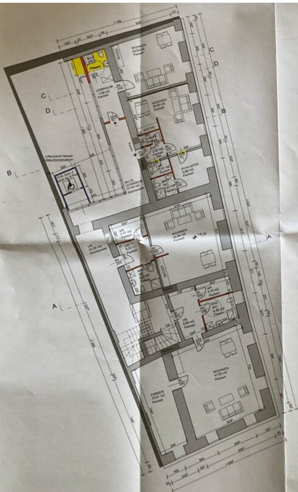
Grundriss 2.Obergeschoss M1:100
