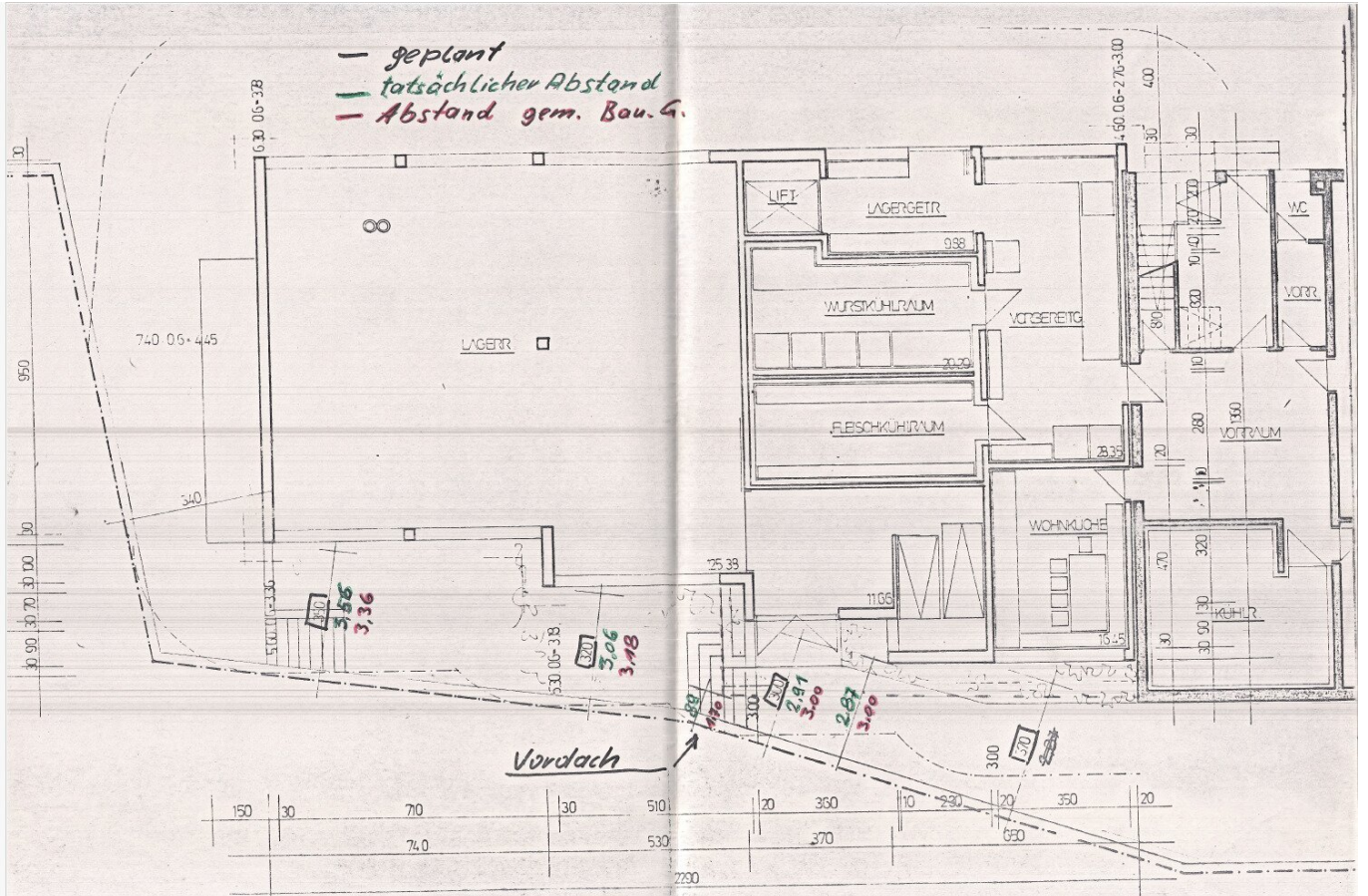
ERDGESCHOSS - GRUNDRISS M 1 : 100
