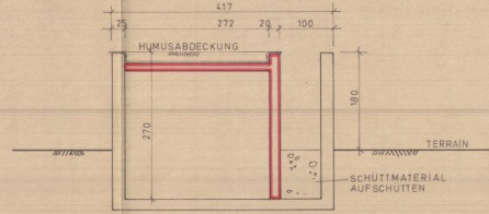
SCHNITT A-A 1:50
