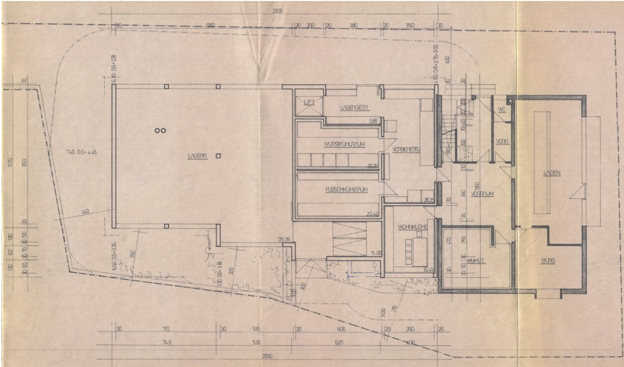
ERDGESCHOSS - GRUNDRISS M 1 : 100
