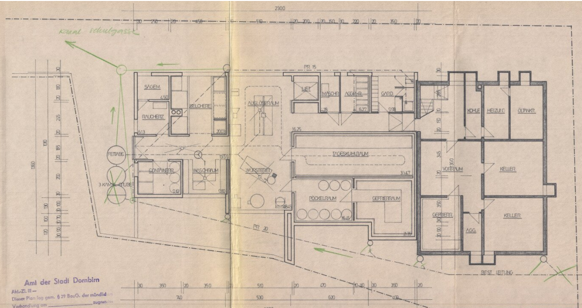
UNTERGESCHOSS-GRUNDRISS M 1 : 100
