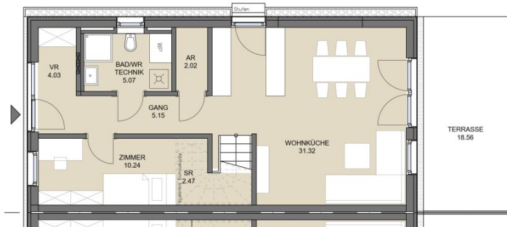
ERDGESCHOSS
